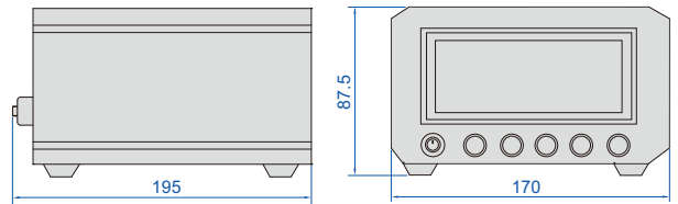
display unit 7131-1A
