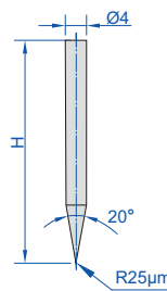
cone stylus
